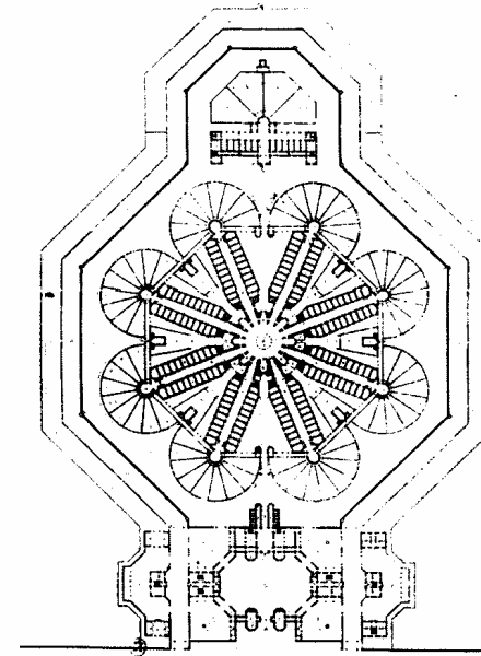
LÁMINA 22. A. Blouet. Proyecto de prisión celular para 585 penados, 1843. Cf. p. 253.
