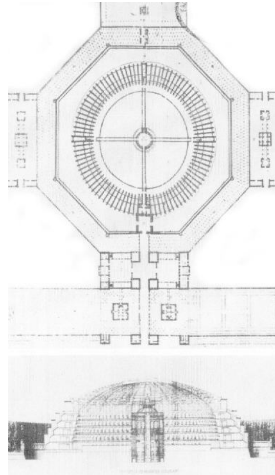
LAMINAS 18 y 19. N. Harou-Romain. Proyectos de penitenciarías, 1840. Cf. p. 253.
